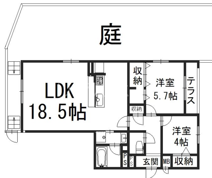
【間取り図】
