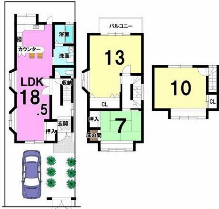
【間取り図】
